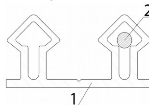
Рисунок 7. ПЭН уплотнителя двери (устанавливается на этапе изготовления во внутреннем контуре уплотнителя двери)
