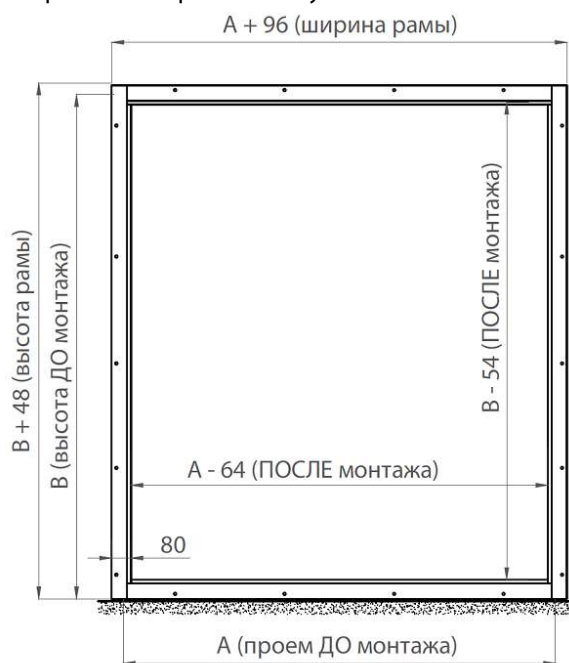
Рисунок 139. Металлическая угловая рама без порога
