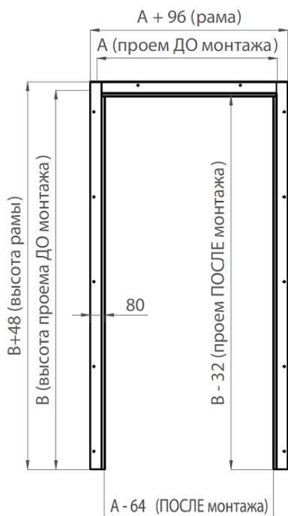
Рисунок 111. Металлическая угловая рама без порога
