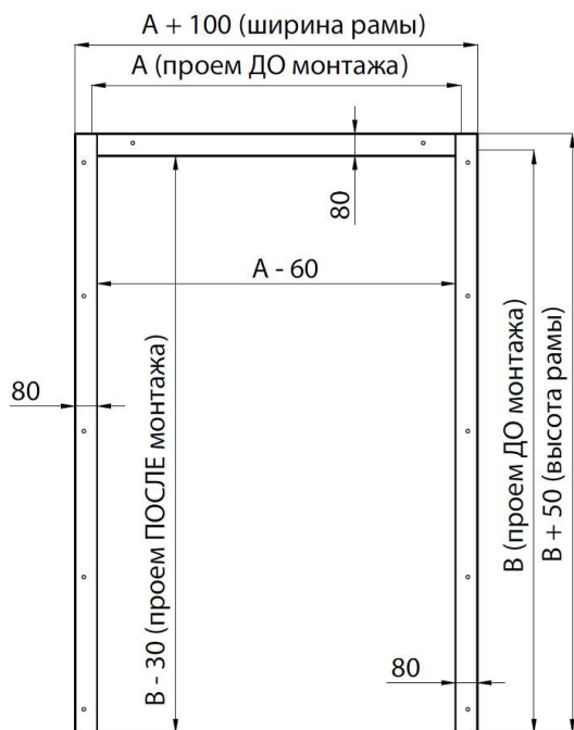
Рисунок 93. Металлическая угловая рама
