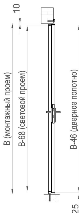
Рисунок 152. Разрез 3-3. ТДД с угловой рамой с порогом 40 мм
