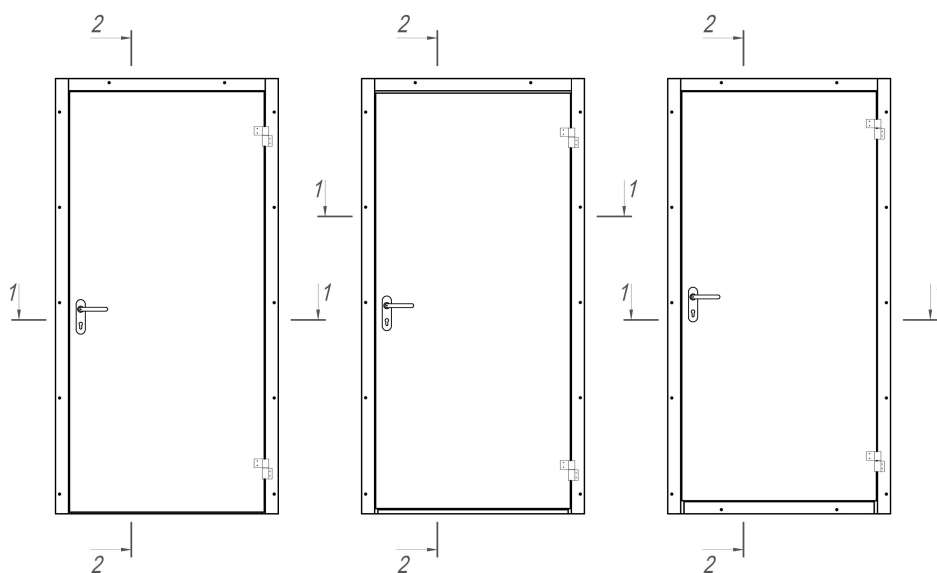
Рисунок 130. ТДО без порога с рамой в обхват проема
