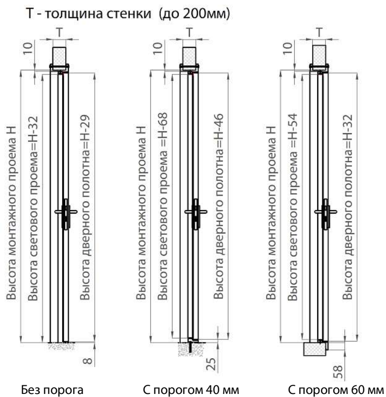
Рисунок 135. Разрез 2-2. ТДО с рамой в обхват проема
