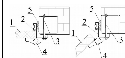
Рисунок 156. Узлы крепления металлической угловой рамы к металлокаркасу (слева — узел 5, справа — узел 6)
