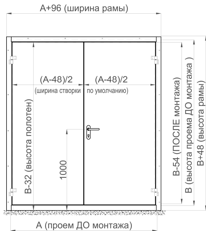
Рисунок 162. ТДД с рамой в обхват проема с порогом 60 мм
