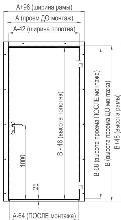
Рисунок 115. ТДО с угловой рамой с порогом 40 мм
