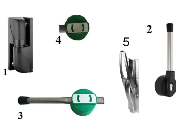
Рисунок 37. Фурнитура РДД серии S (Stuv): 1 — дверная металлическая петля с регулировками в трех плоскостях, 2 — наружная поворотная ручка со встроенным замком, 3 — внутренняя поворотная ручка аварийного открывания, 4 — дополнительный затвор для дверей высотой более 2400 мм, 5 — ручка дополнительной створки
