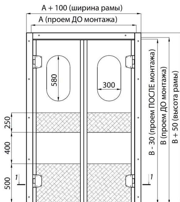
Рисунок 94. МДД с угловой рамой
