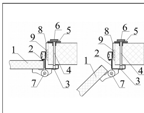
Рисунок 151. Разрез 2-2. ТДД с угловой рамой без порога
