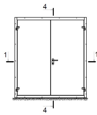
Рисунок 147. Местоположение разрезов на ТДД с порогом 60 мм
