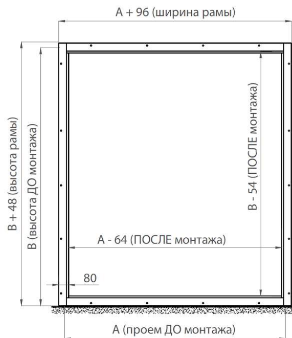
Рисунок 159. Металлическая угловая рама с порогом 60 мм
