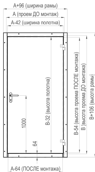
Рисунок 116. ТДО с угловой рамой с порогом 60 мм
