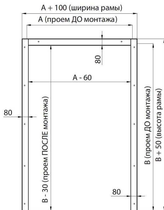
Рисунок 104. Металлическая рама, устанавливаемая в обхват проема
