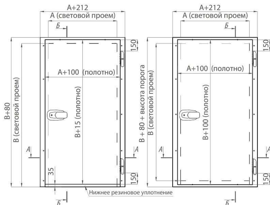
Рисунок 20. Распашные двери РДО с накладной металлической рамой (слева — без порога, справа — с порогом)
