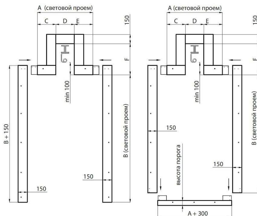
Рисунок 52. Металлическая накладная рама для проемов с технологическим монорельсом (слева — без порога, справа — с порогом)
