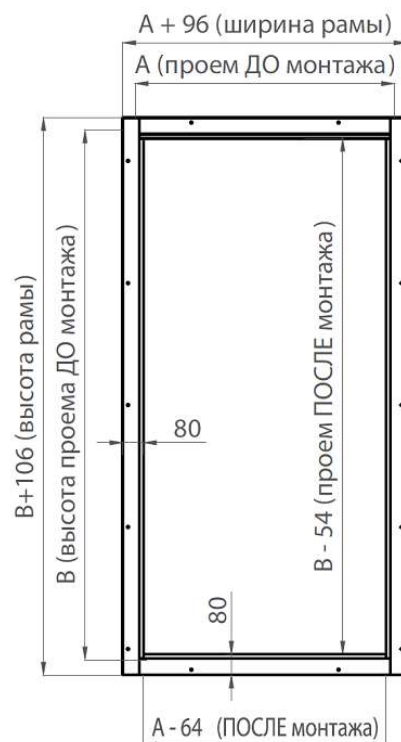
Рисунок 113: Металлическая угловая рама с порогом 60 мм
