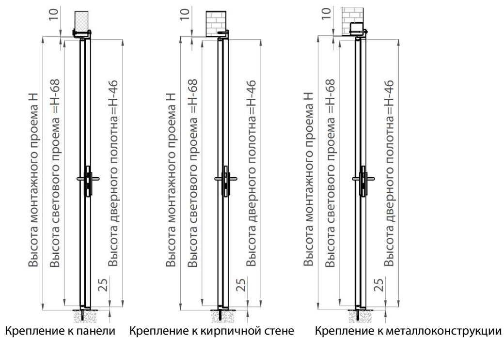
Рисунок 122. Разрез 3-3. ТДО с угловой рамой с порогом 40 мм
