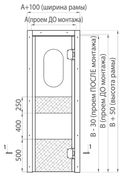
Рисунок 79. МДО с угловой рамой
