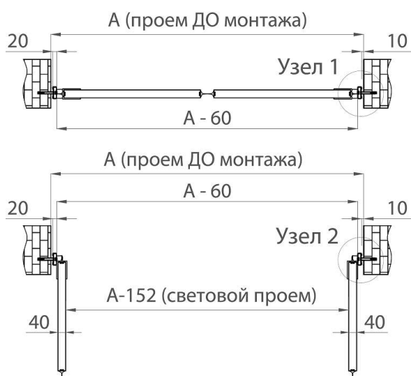
Рисунок 101. Разрез 1-1. Крепление к кирпичной стене (с плоским отбойником)
