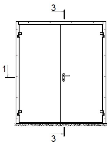
Рисунок 164. Местоположение разрезов на ТДД с порогом 40 мм
