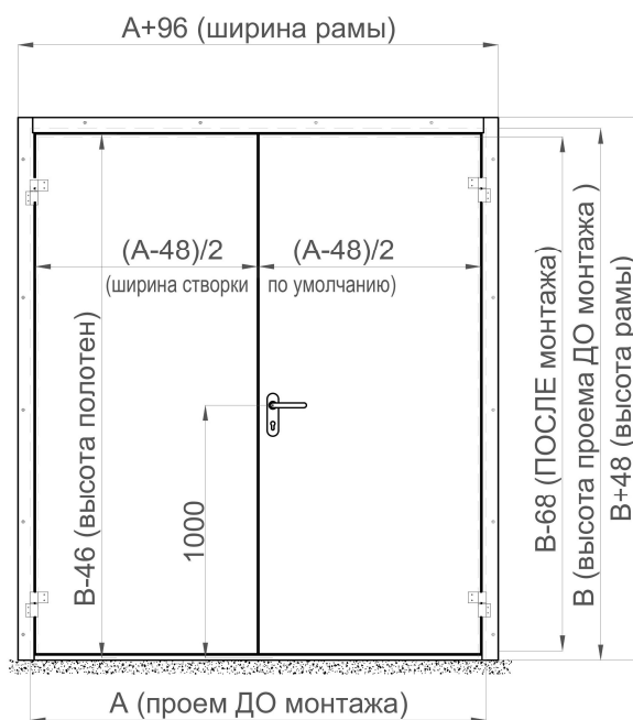
Рисунок 143. ТДД с угловой рамой с порогом 40 мм
