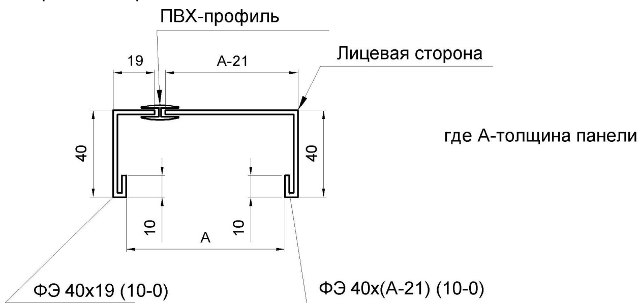
Рисунок 1. Профиль для обрамления светового проема в сэндвич-панелях (чертеж с размерами)
