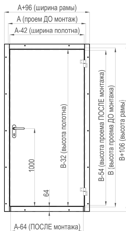
Рисунок 132. ТДО с порогом 60 с рамой в обхват проема
