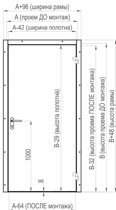
Рисунок 114. ТДО с угловой рамой без порога
