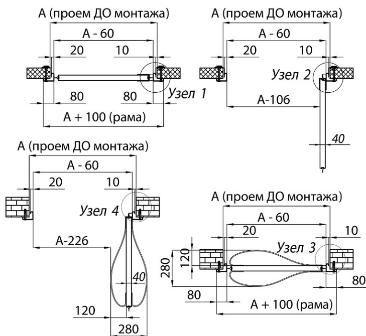
Рисунок 80. Разрез 1-1: сверху — крепление к панели (вариант с плоским отбойником), внизу — крепление к кирпичной стене (вариант с изогнутым отбойником)
