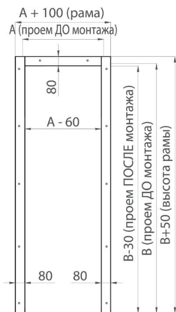
Рисунок 78. Металлическая угловая рама
