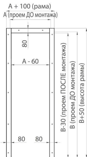
Рисунок 87. Металлическая рама, устанавливаемая в обхват проема
