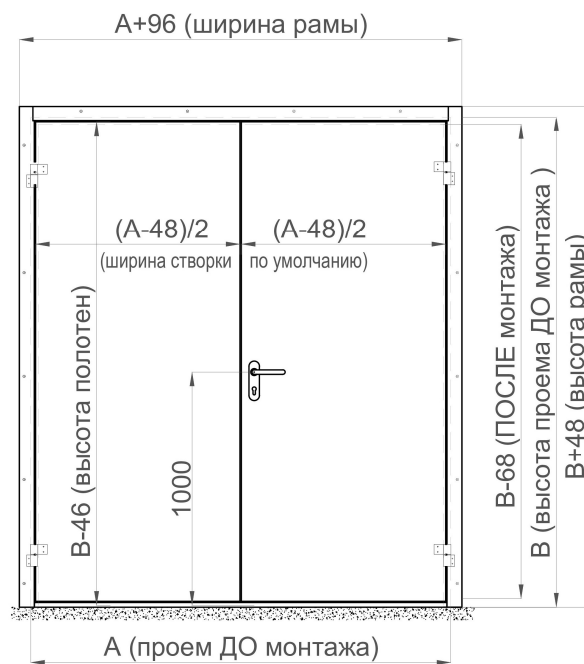
Рисунок 161. ТДД с рамой в обхват проема с порогом 40 мм
