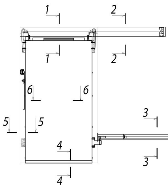
Рисунок 64. Металлическая накладная рама для ОД легкой серии (слева — вариант без порога, справа — вариант с порогом)
