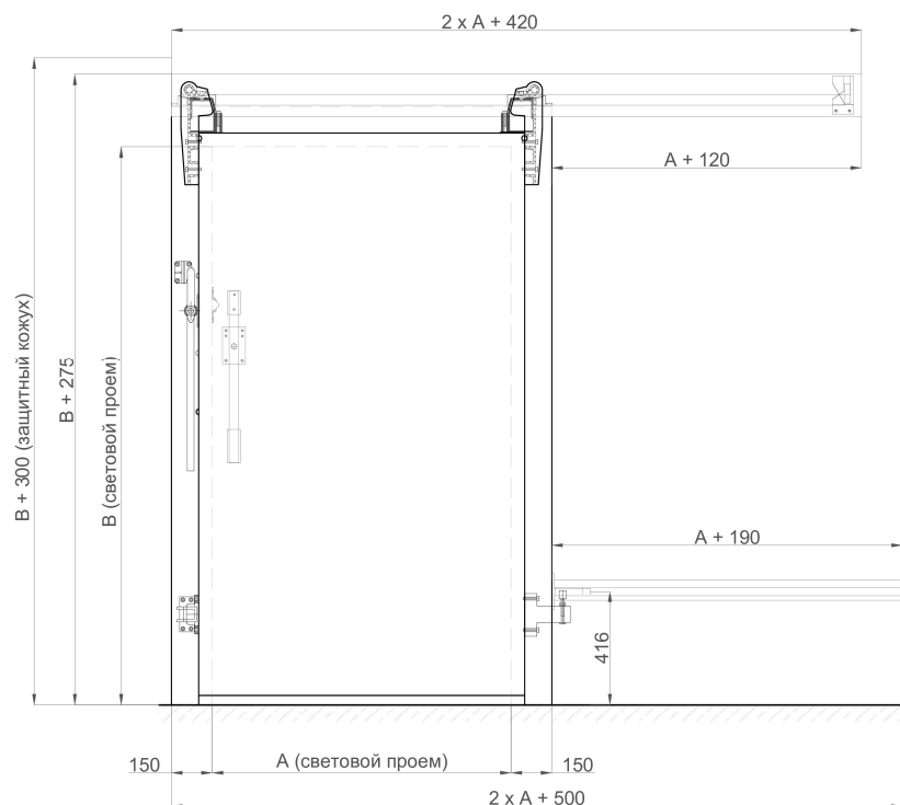
Рисунок 51. Откатная дверь ОД тяжелой серии, укомплектованная накладной металлической рамой, а также нижней и верхней направляющими для стандартных проемов
