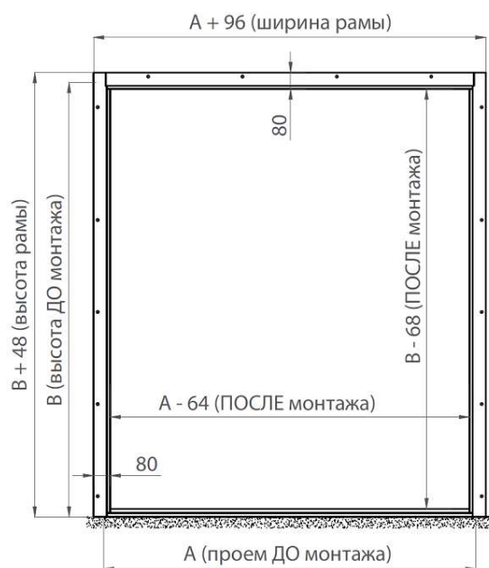
Рисунок 140. Металлическая угловая рама с порогом 40 мм
