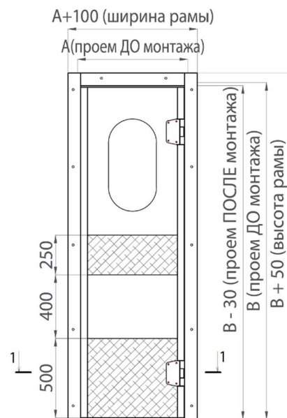
Рисунок 88. МДО с металлической рамой, устанавливаемой в обхват проема
