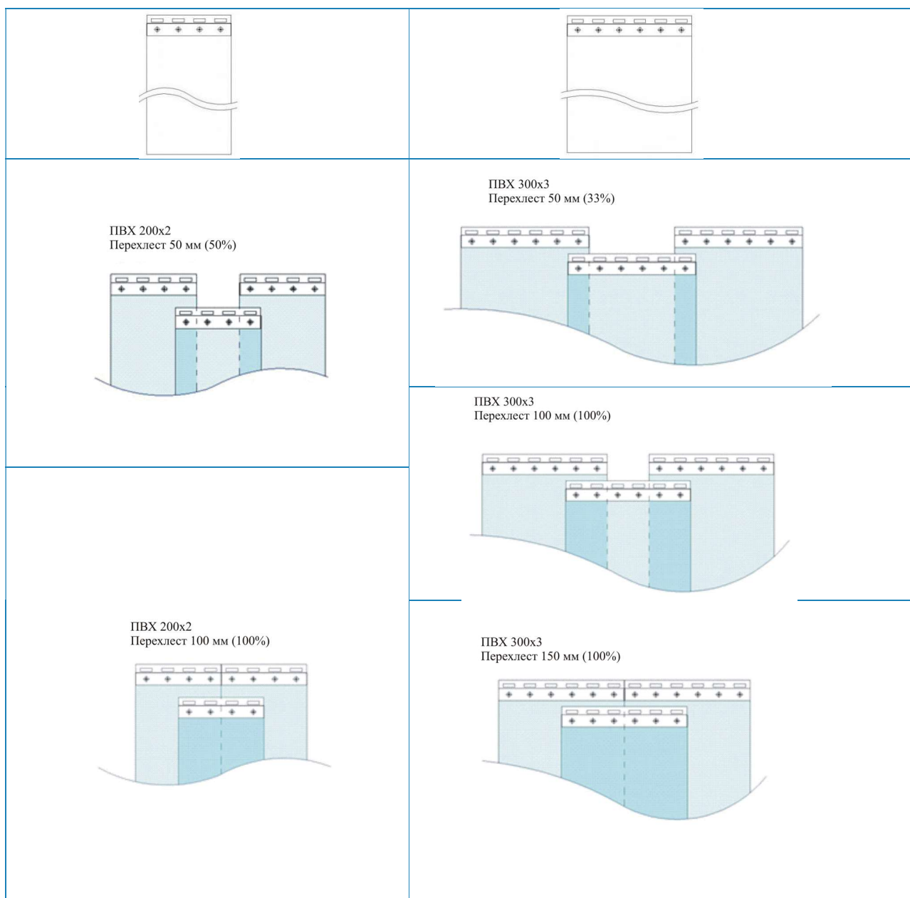
Рисунок 15. ПВХ-ленты шириной 200 и 300 мм с разным перехлестом
