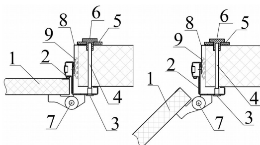
Рисунок 123. Разрез 4-4. ТДО с угловой рамой с порогом 60 мм
