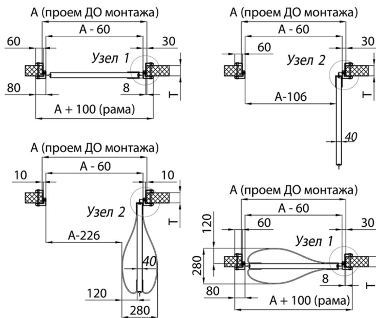
Рисунок 89. Разрез 1-1. Крепление металлической рамы в обхват (вверху — вариант с плоским отбойником, внизу — вариант с изогнутым отбойником, Т — толщина стенки (не более 200 мм))
