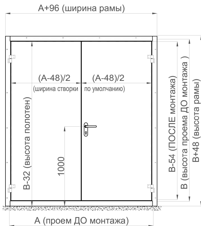
Рисунок 144. ТДД с угловой рамой с порогом 60 мм
